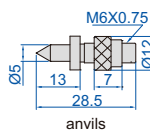
anvils
