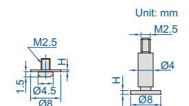
1148-P101 and 1148-P102
